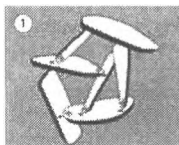
1 Leire med saltholdig porevann: Åpen, men stabil kornstruktur. Saltet binder partiklene sammen.
