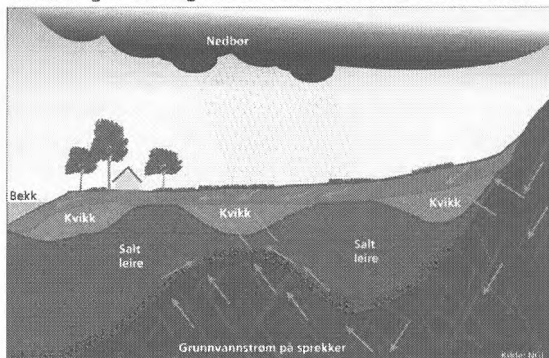
Utvasking av salt og dannelse av kvikkleire i marin leire
