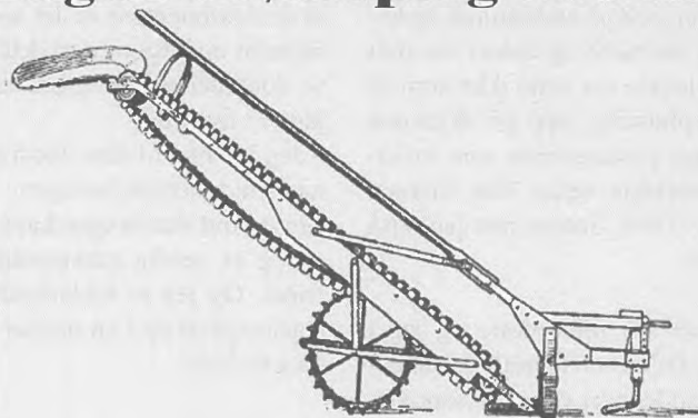
Fig. 35. Engens grøfteplog.
